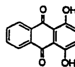
QUINIZARIN
